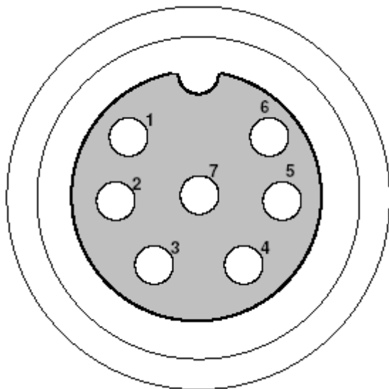
Vorderansicht Kabeldose am Verbindungskabel
