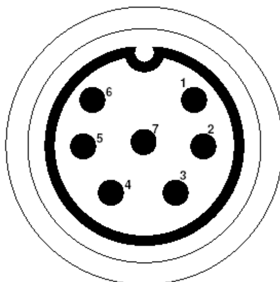
Vorderansicht Kabelstecker an der Wiegeanzeige
